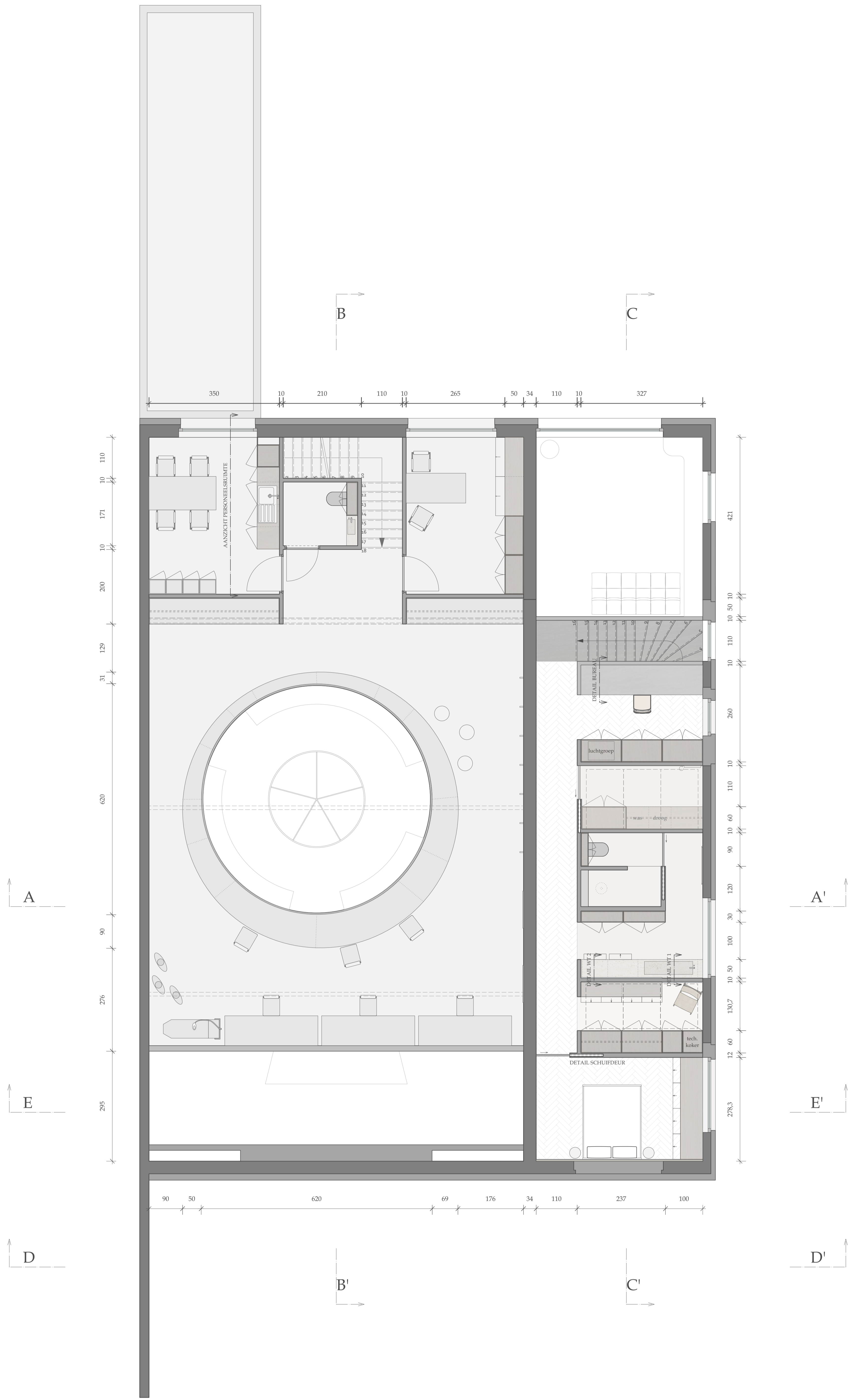
GRONDPLAN V1 - 1/50
