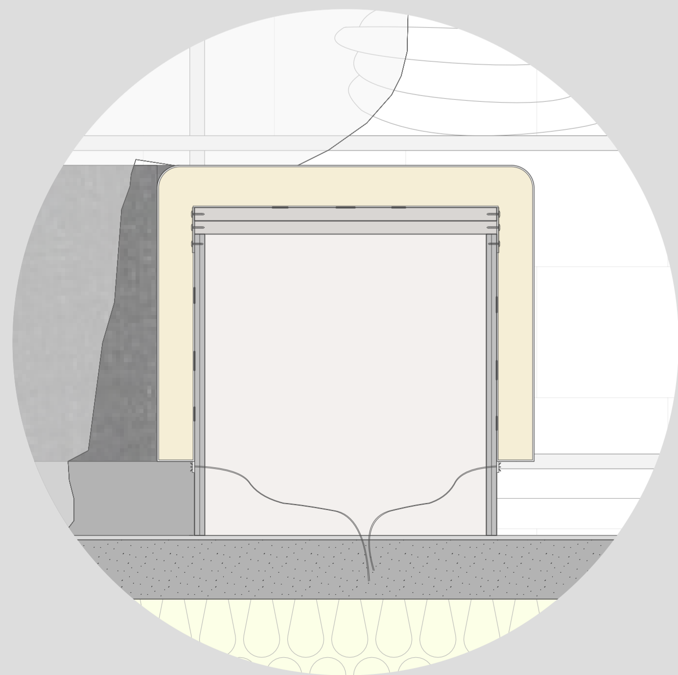
DETAIL ZITBANK - 1/5
