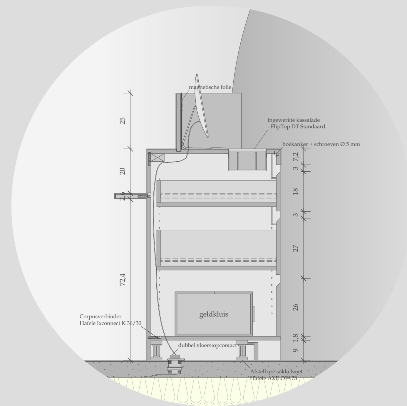
DETAIL KASSA - 1/10
