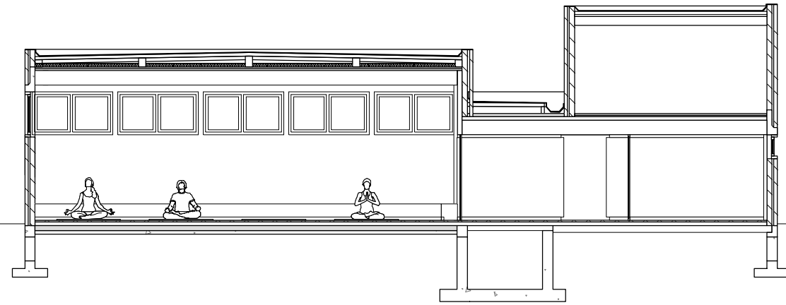
SNEDE CC'
