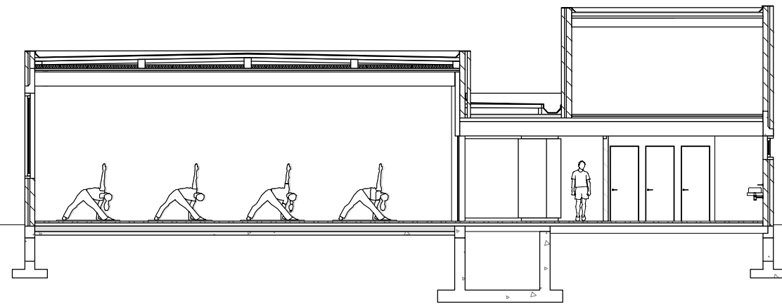
SNEDE DD'
